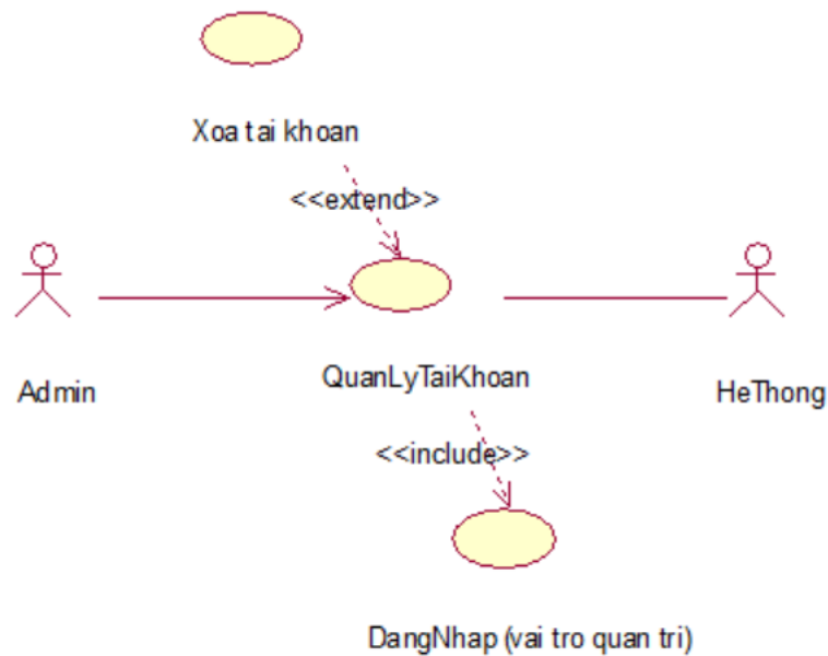
Hình 2.13. Mô hình hóa chức năng Quản lý tài khoản
