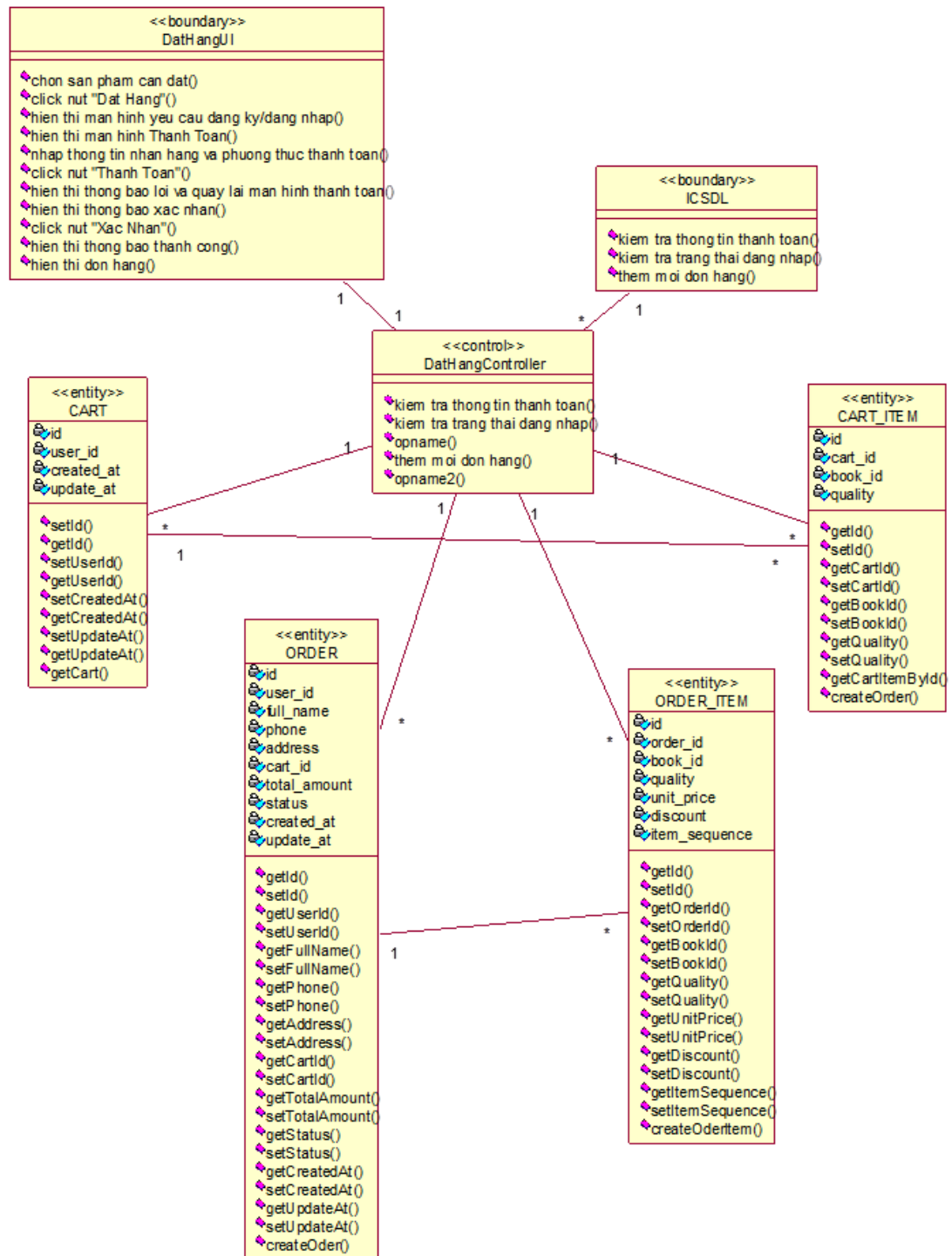
Hình 3.24. Biểu đồ lớp (VOPC) chức năng “Đặt hàng”
