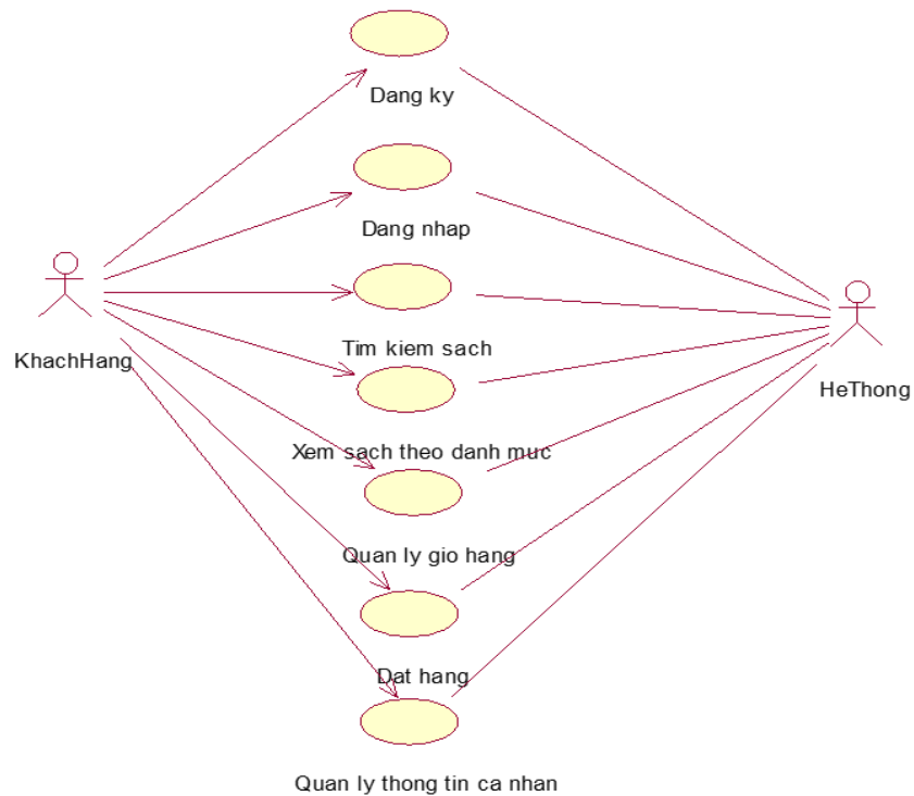
Hình 2.3. Biểu đồ Use case phía Khách Hàng
