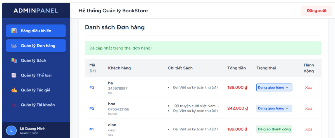
Hình 5.21. Kết quả test case 3 “Quản lý đơn hàng”
