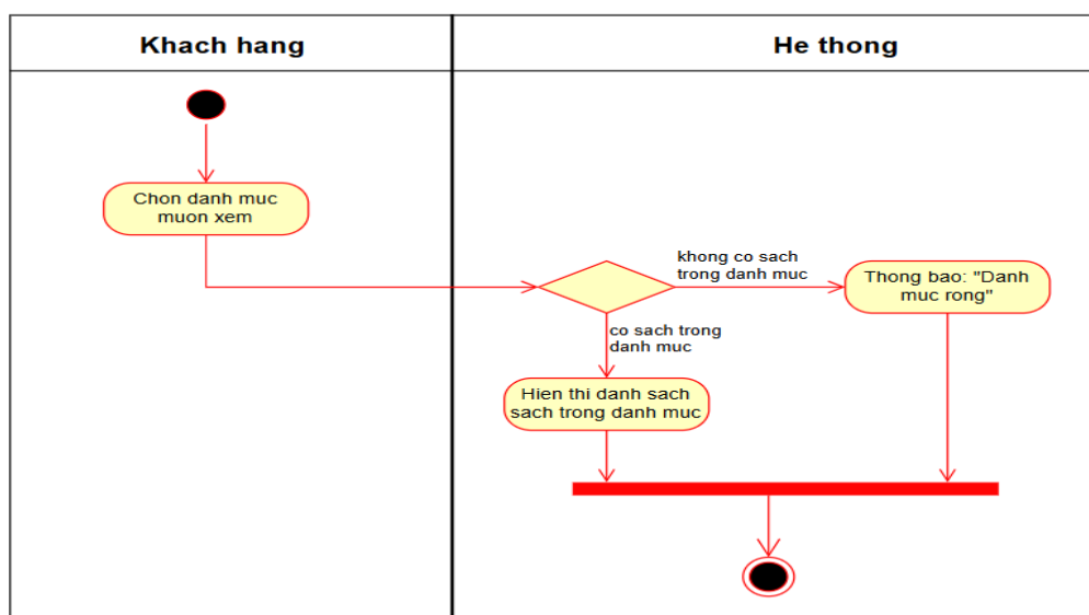
Hình 3.14. Biểu đồ hoạt động chức năng “Xem sách theo danh mục”
