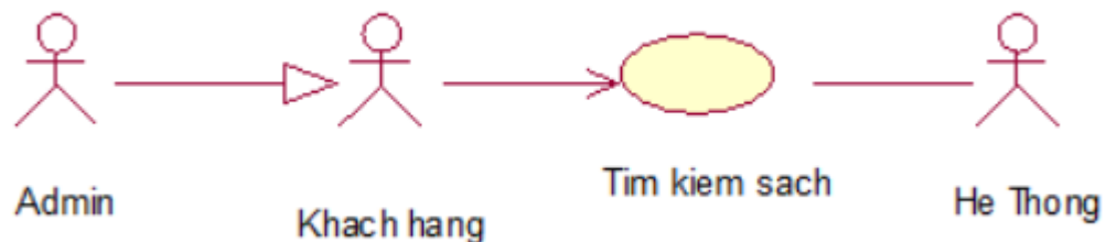
Hình 2.7. Mô hình hóa chức năng Tìm kiếm sách
