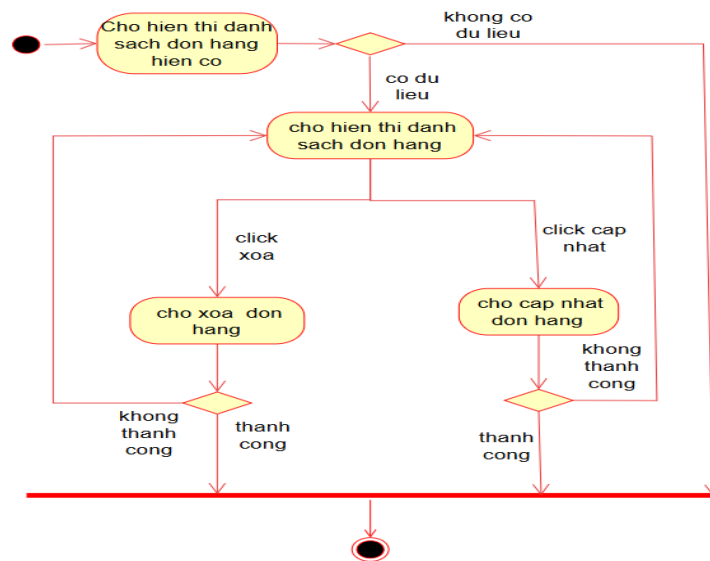
Hình 3.37. Biểu đồ trạng thái chức năng “Quản lý đơn hàng”
