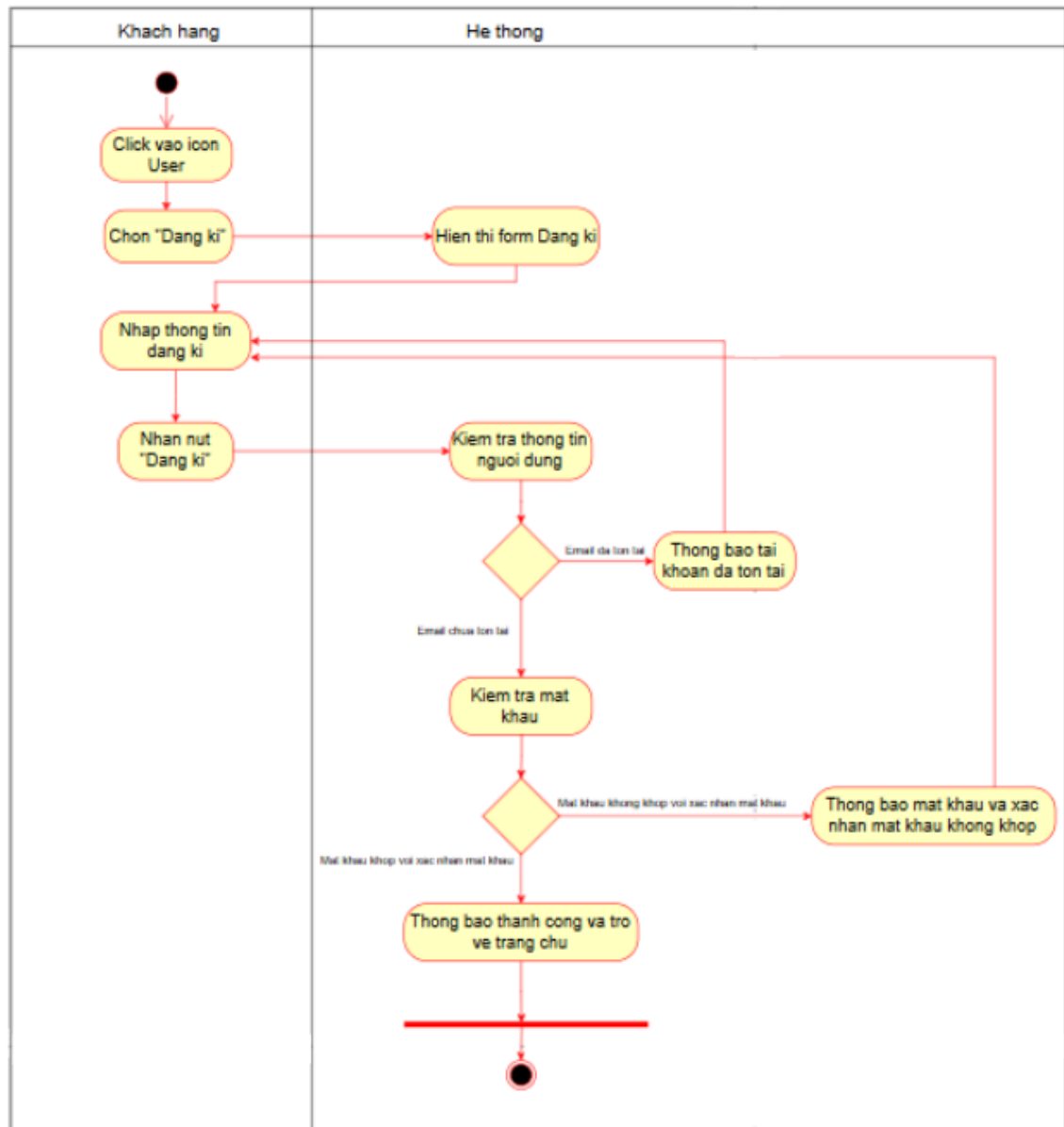
Hình 3.2. Biểu đồ hoạt động chức năng “Đăng ký”
