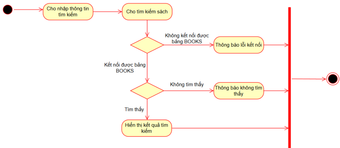
Hình 3.9. Biểu đồ trạng thái chức năng “Tìm kiếm sách”
