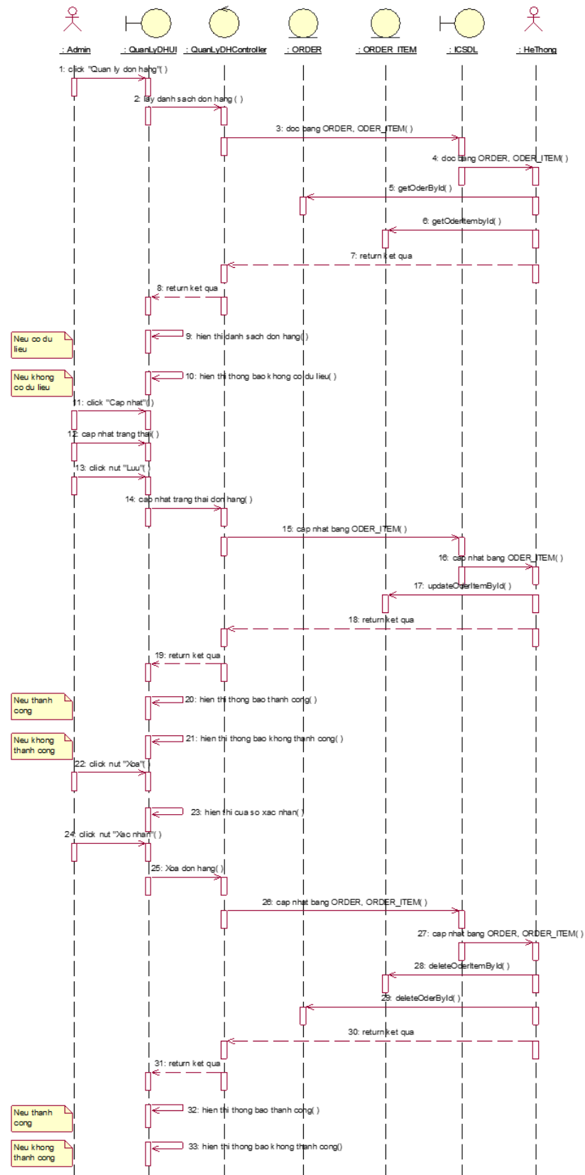
Hình 3.39. Biểu đồ trình tự chức năng “Quản lý đơn hàng”
