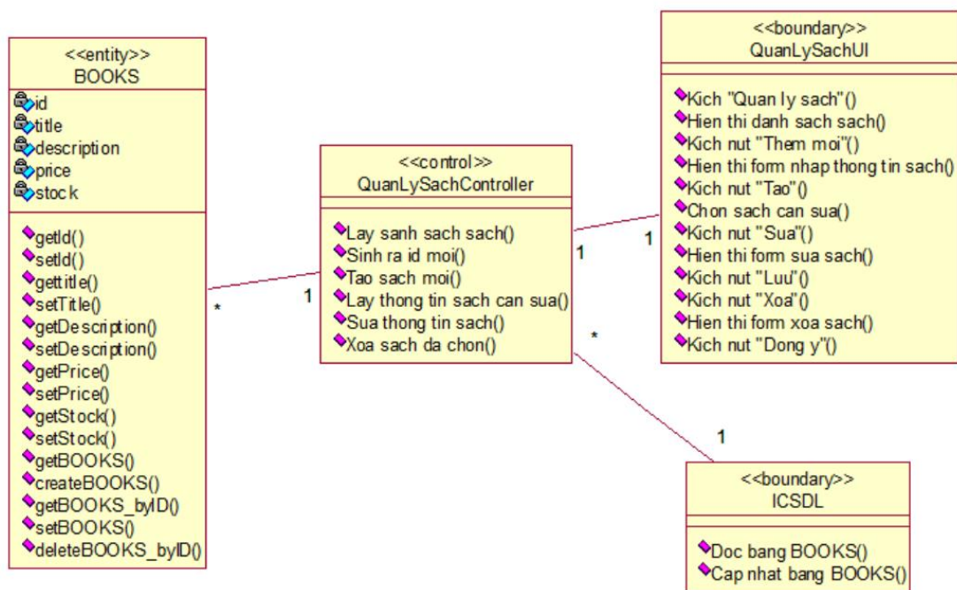
Hình 3.32. Biểu đồ lớp (VOPC) chức năng “Quản lý sách”
