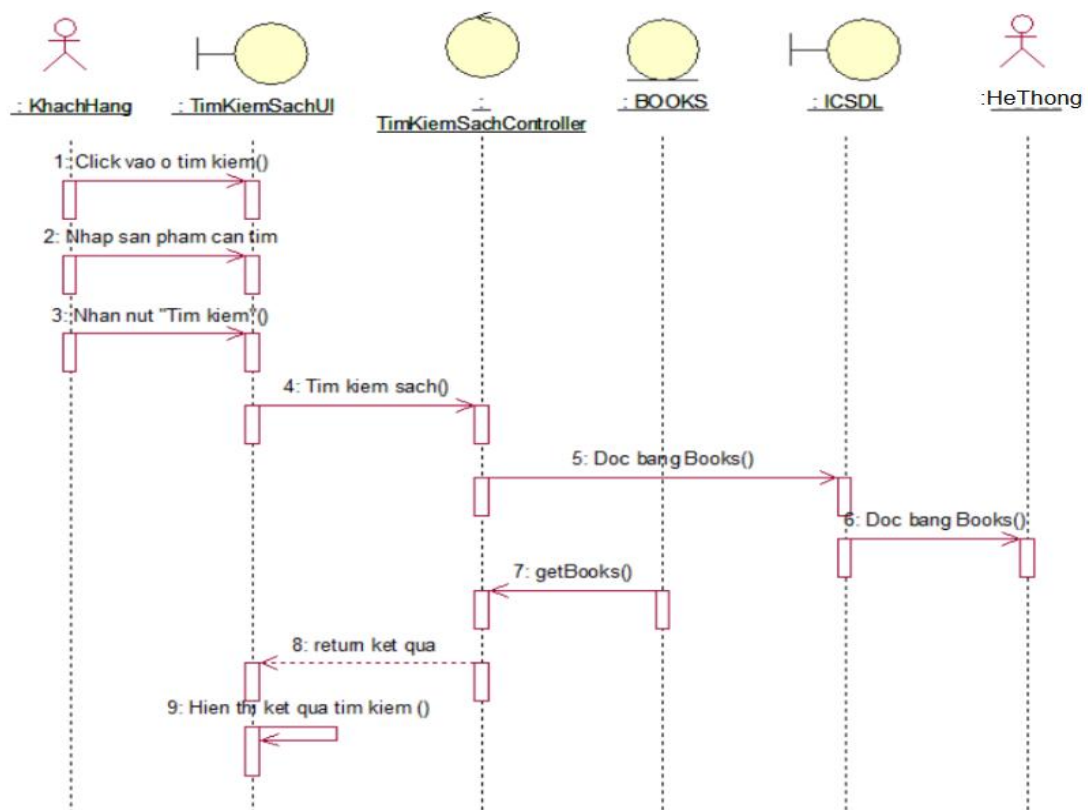
Hình 3.11. Biểu đồ trình tự chức năng “Tìm kiếm sách”
