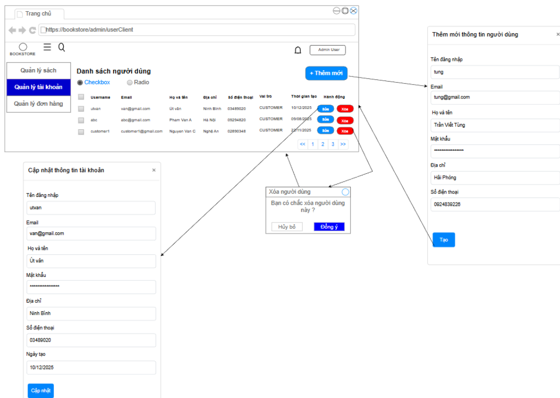
Hình 3.51. Mô phỏng màn hình “Quản lý tài khoản”
