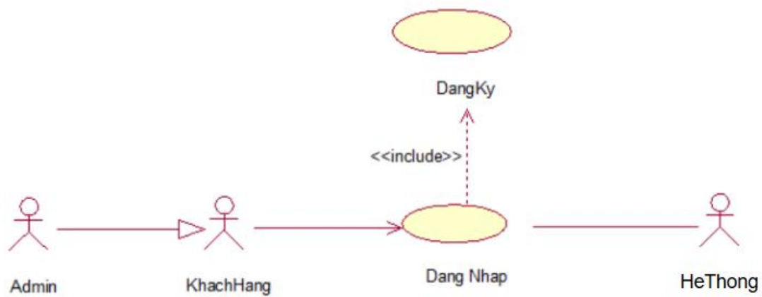
Hình 2.6. Mô hình hóa chức năng Đăng nhập
