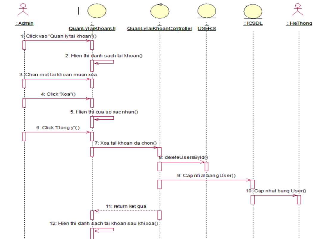
Hình 3.35. Biểu đồ trình tự chức năng “Quản lý tài khoản”
