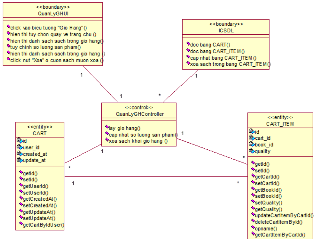
Hình 3.20. Biểu đồ lớp (VOPC) chức năng “Quản lý giỏ hàng”
