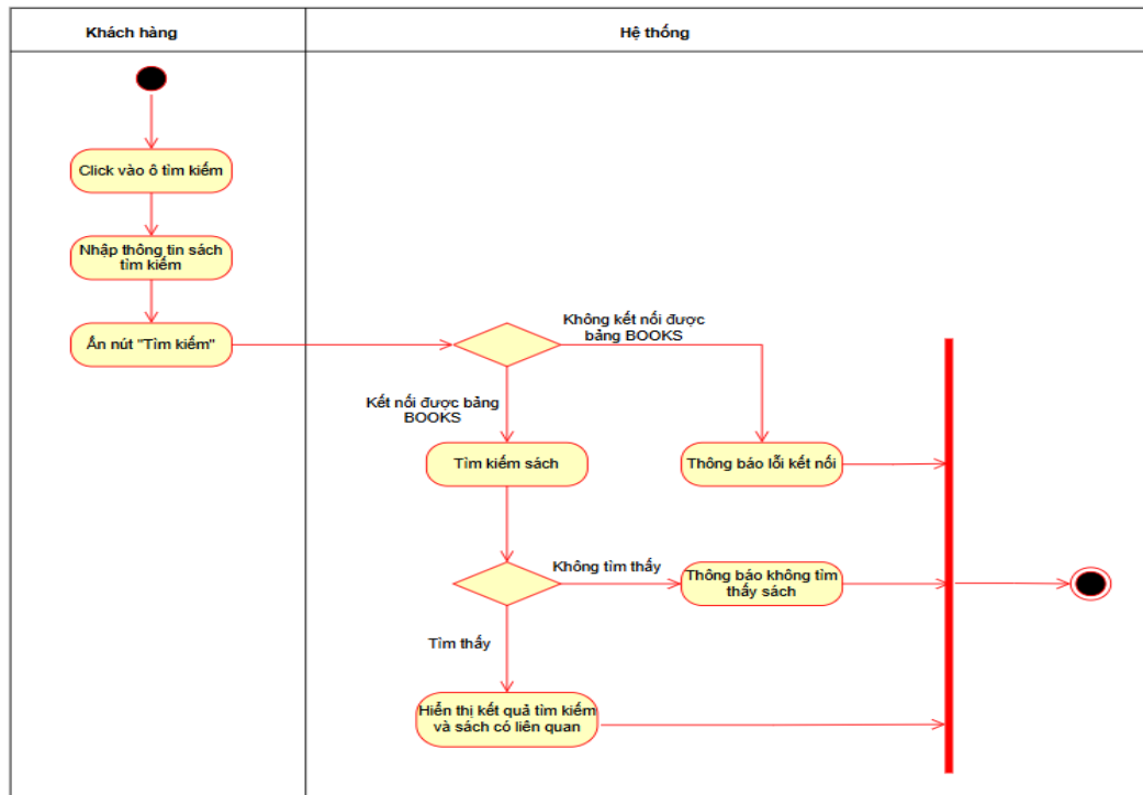
Hình 3.10. Biểu đồ hoạt động chức năng “Tìm kiếm sách”
