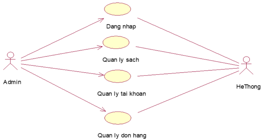
Hình 2.4. Biểu đồ Use case phía Quản trị
