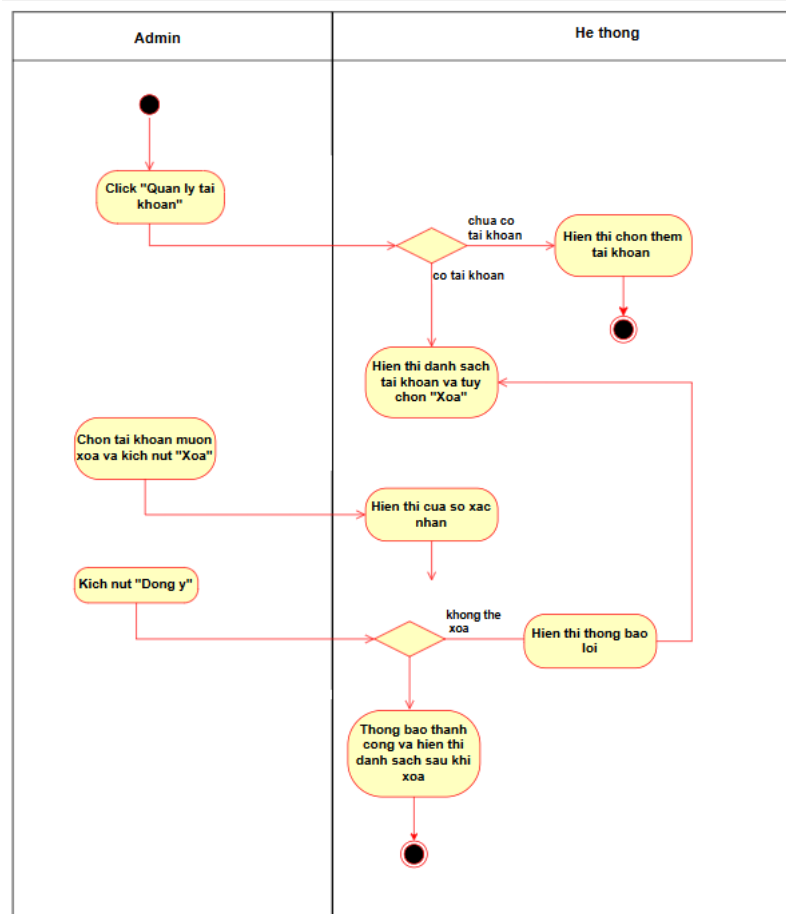
Hình 3.34. Biểu đồ hoạt động chức năng “Quản lý tài khoản”
