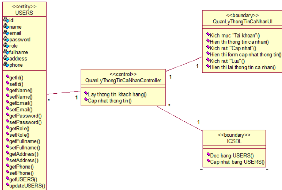
Hình 3.28. Biểu đồ lớp (VOPC) chức năng “Quản lý thông tin cá nhân”
