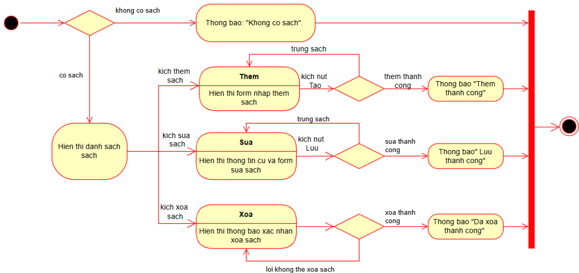
Hình 3.29. Biểu đồ trạng thái chức năng “Quản lý sách”
