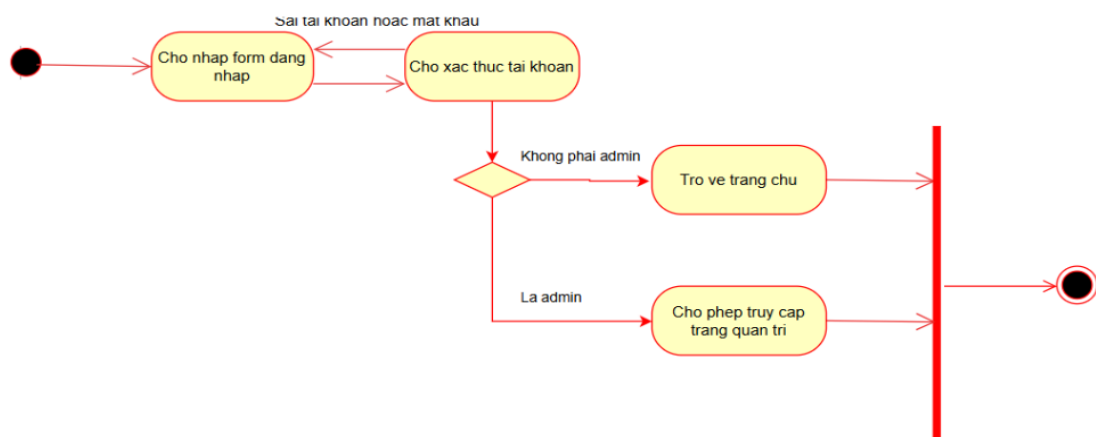
Hình 3.5. Biểu đồ trạng thái chức năng “Đăng nhập”
