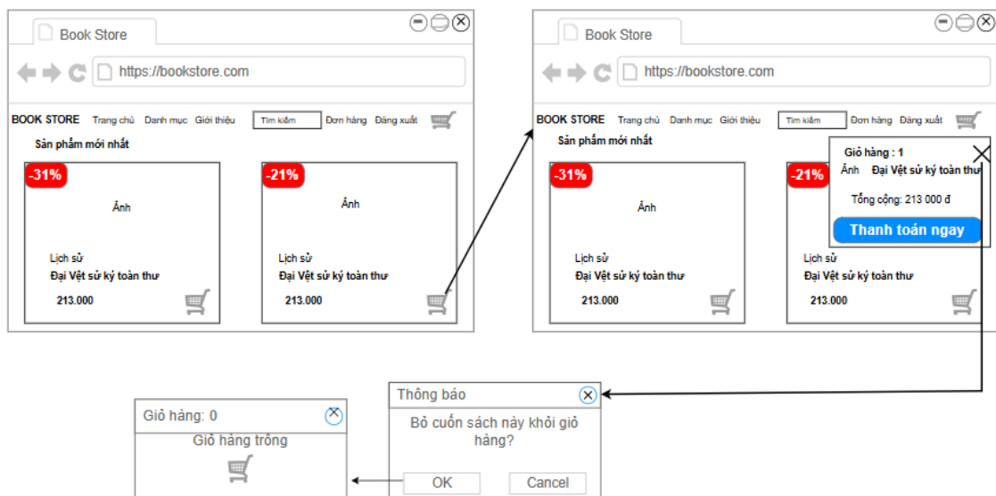
Hình 3.47. Mô phỏng màn hình “Quản lý giỏ hàng”
