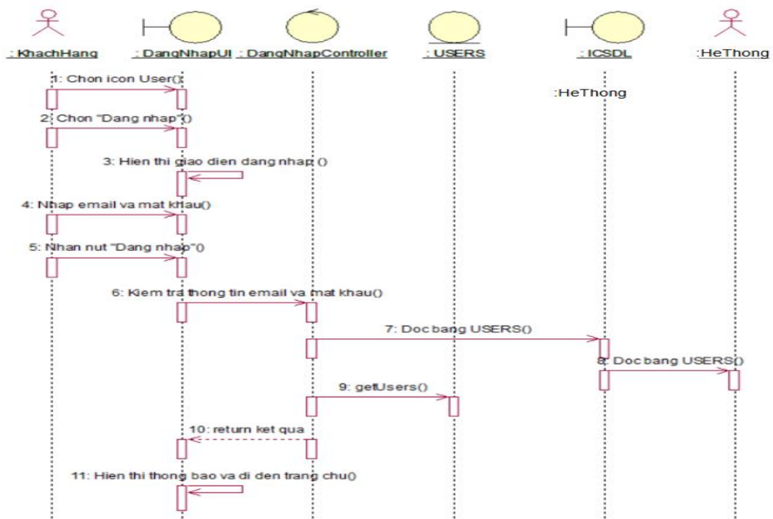
Hình 3.7. Biểu đồ trình tự chức năng “Đăng nhập”
