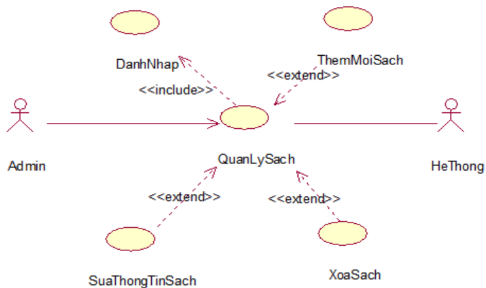
Hình 2.12. Mô hình hóa chức năng Quản lý sách
