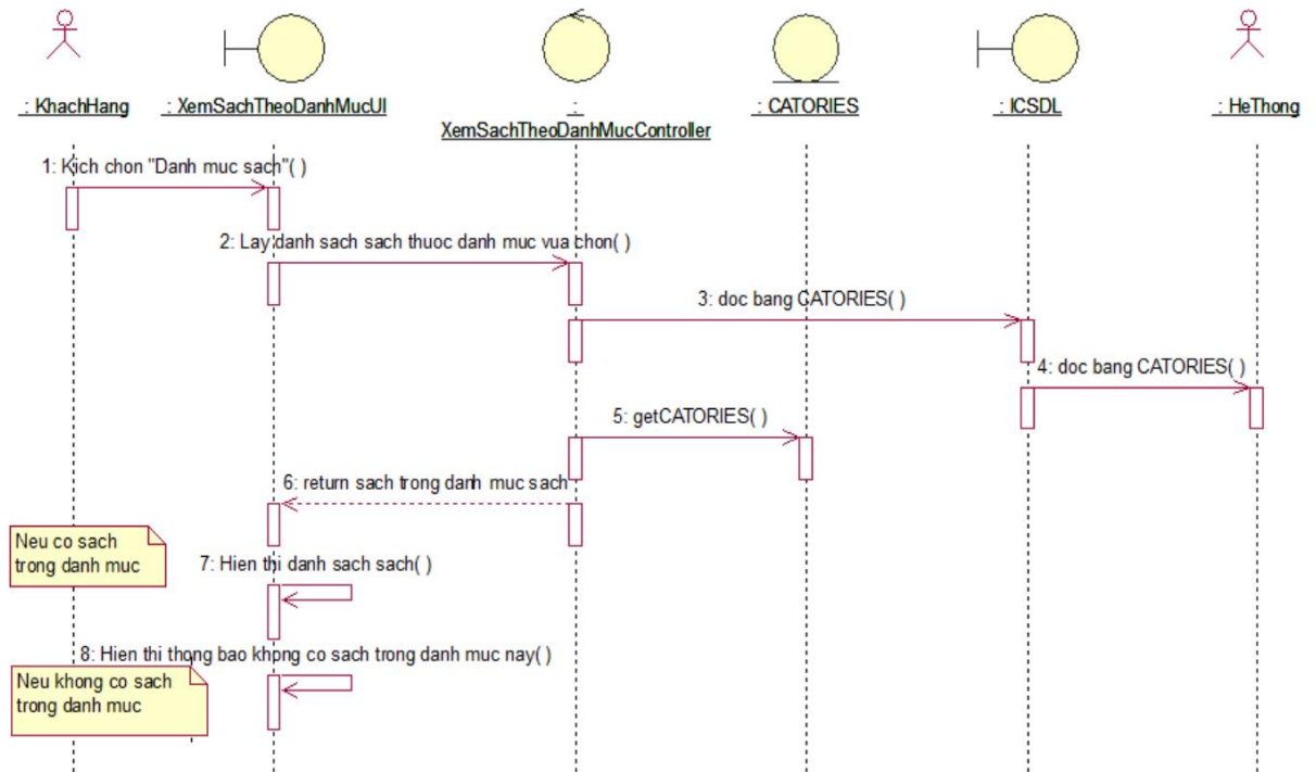
Hình 3.15. Biểu đồ trình tự chức năng “Xem sách theo danh mục”
