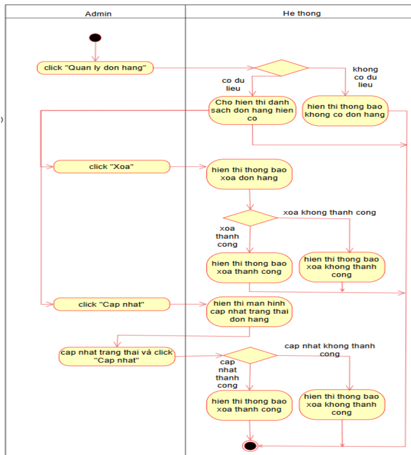
Hình 3.38. Biểu đồ hoạt động chức năng “Quản lý đơn hàng”
