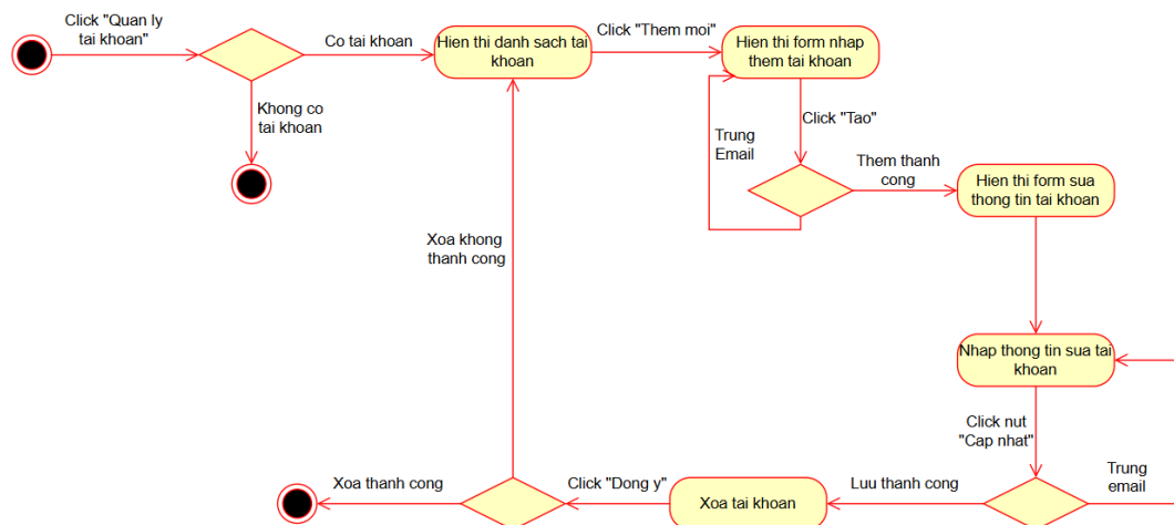
Hình 3.33. Biểu đồ trạng thái chức năng “Quản lý tài khoản”
