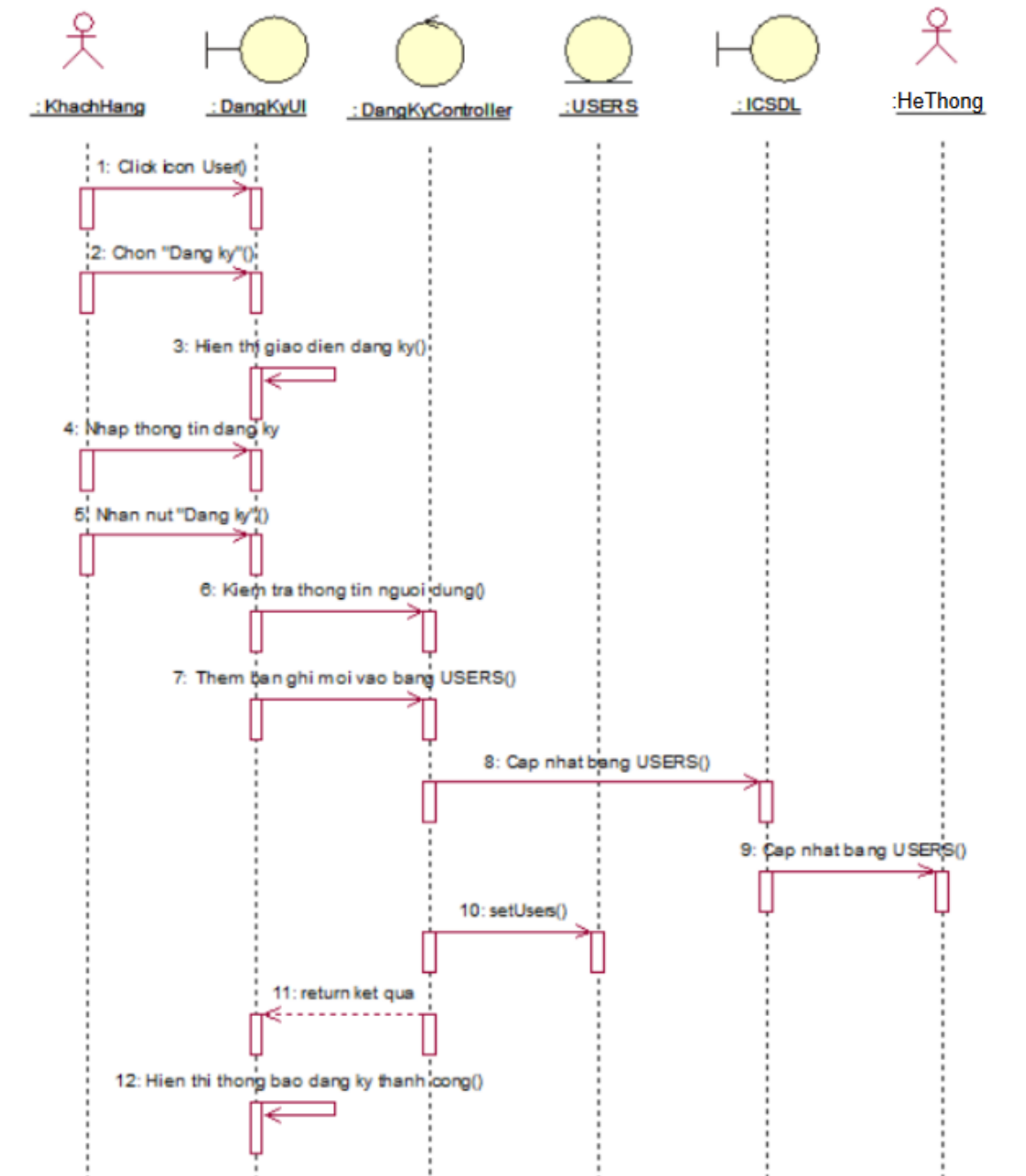
Hình 3.3. Biểu đồ trình tự chức năng “Đăng ký”
