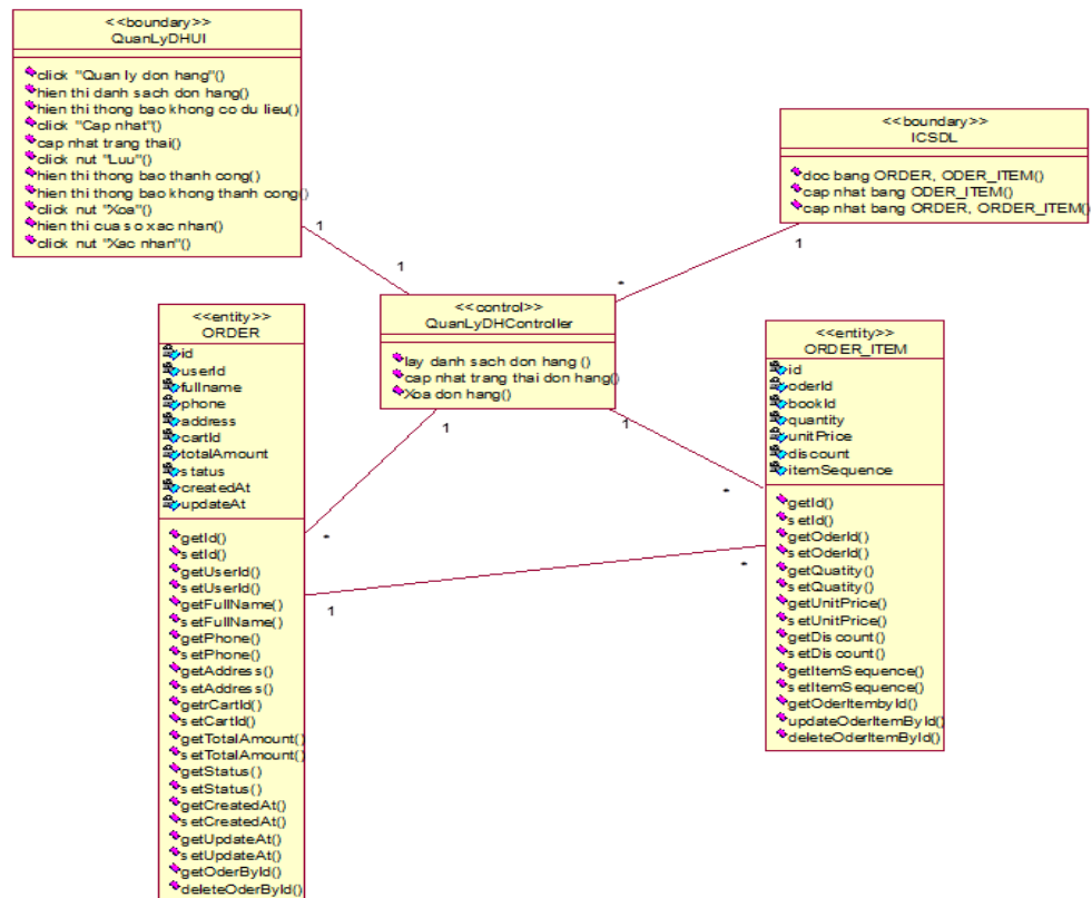
Hình 3.40. Biểu đồ lớp (VOPC) chức năng “Quản lý đơn hàng”
