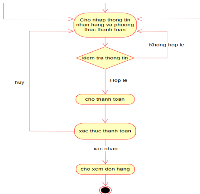
Hình 3.21. Biểu đồ trạng thái chức năng “Đặt hàng”
