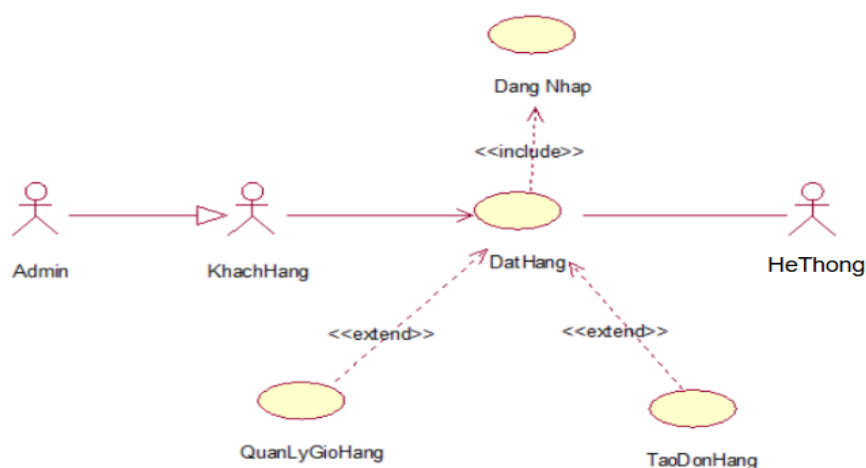
Hình 2.10. Mô hình hóa chức năng Đặt hàng
