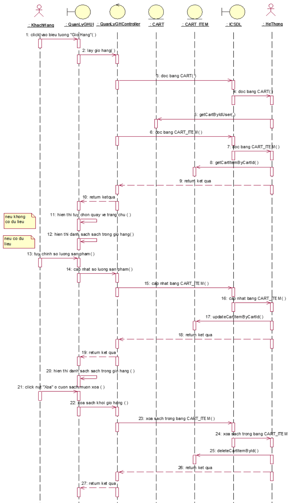
Hình 3.19. Biểu đồ trình tự chức năng “Quản lý giỏ hàng”
