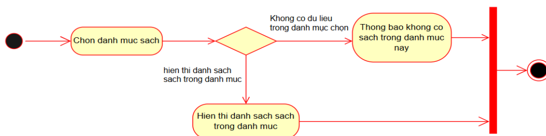
Hình 3.13. Biểu đồ trạng thái chức năng “Xem sách theo danh mục”
