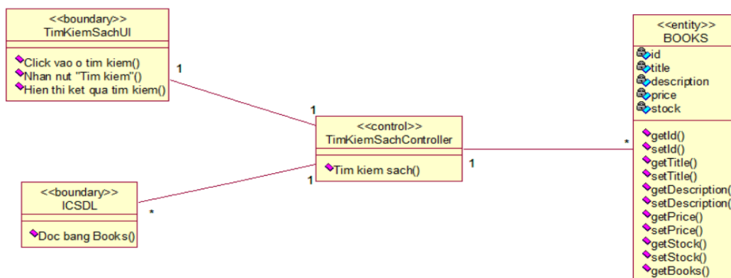
Hình 3.12. Biểu đồ lớp (VOPC) chức năng “Tìm kiếm sách”
