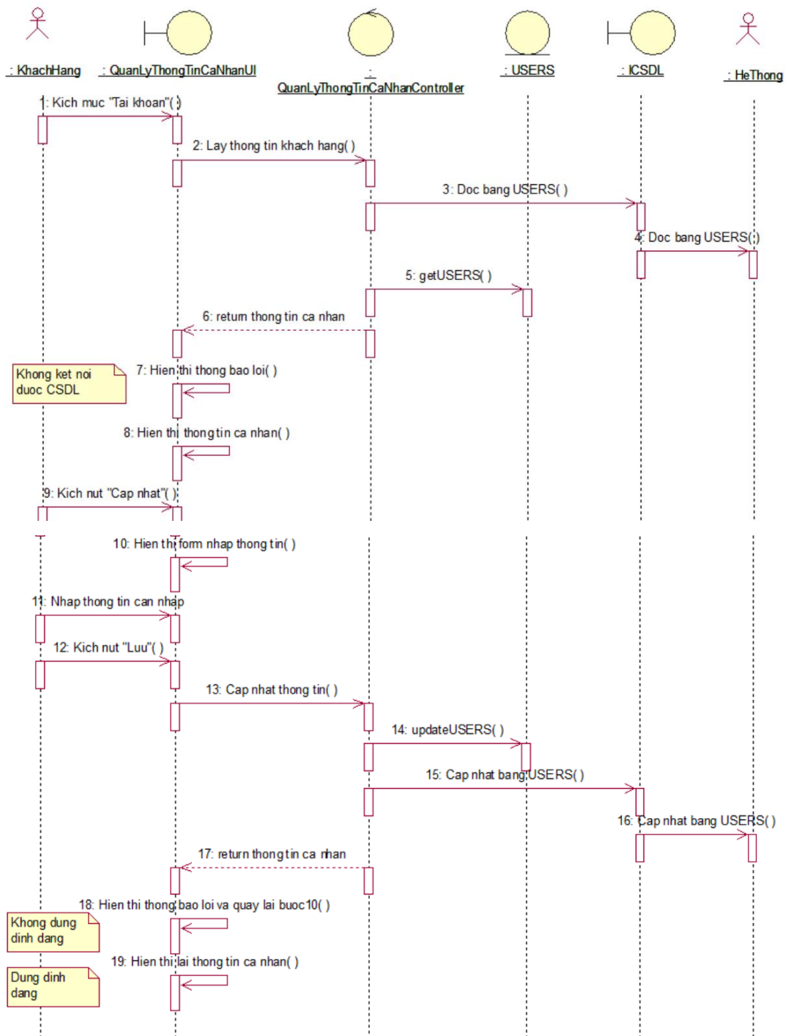
Hình 3.27. Biểu đồ trình tự chức năng “Quản lý thông tin cá nhân”
