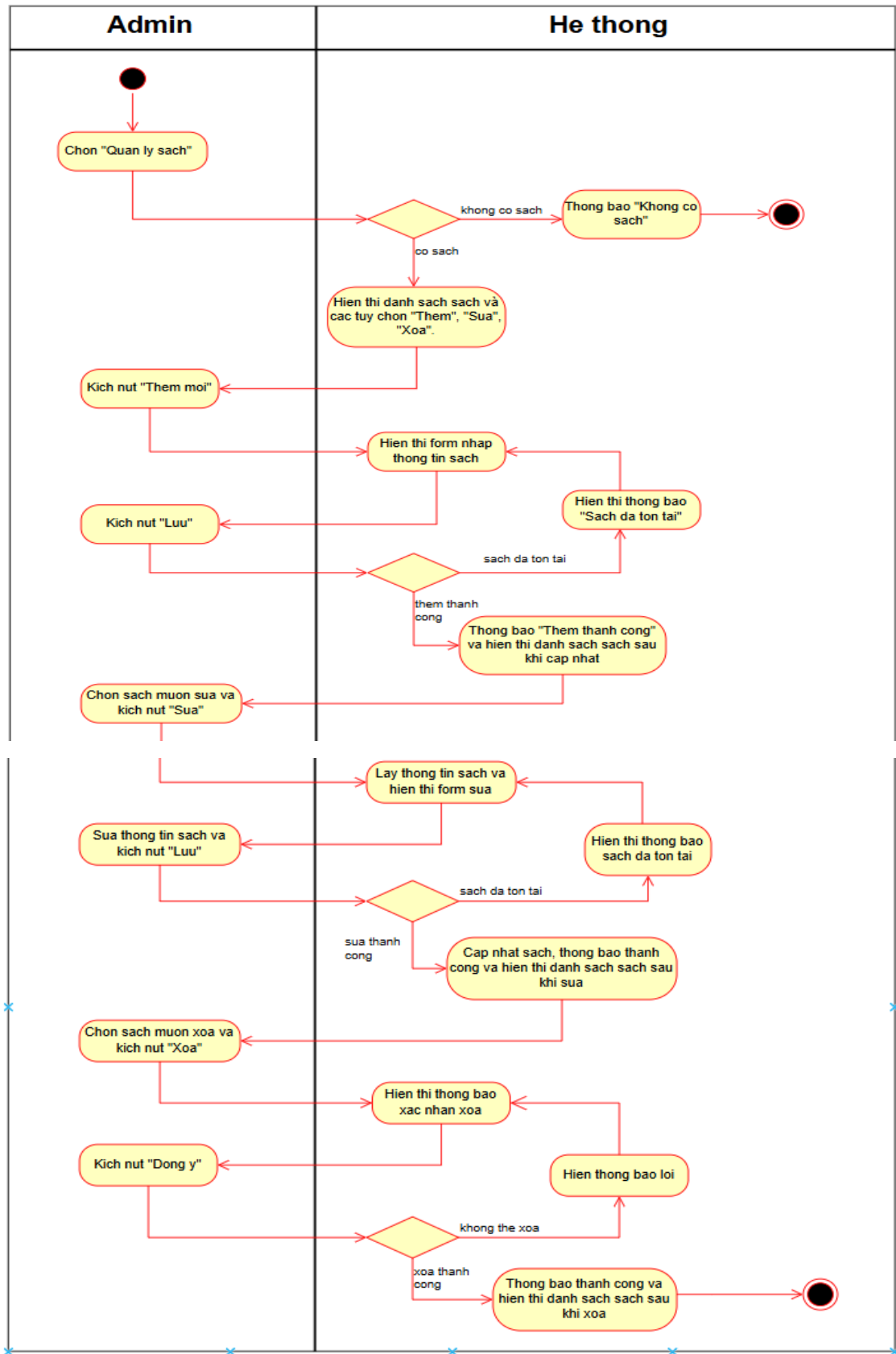
Hình 3.30. Biểu đồ hoạt động chức năng “Quản lý sách”
