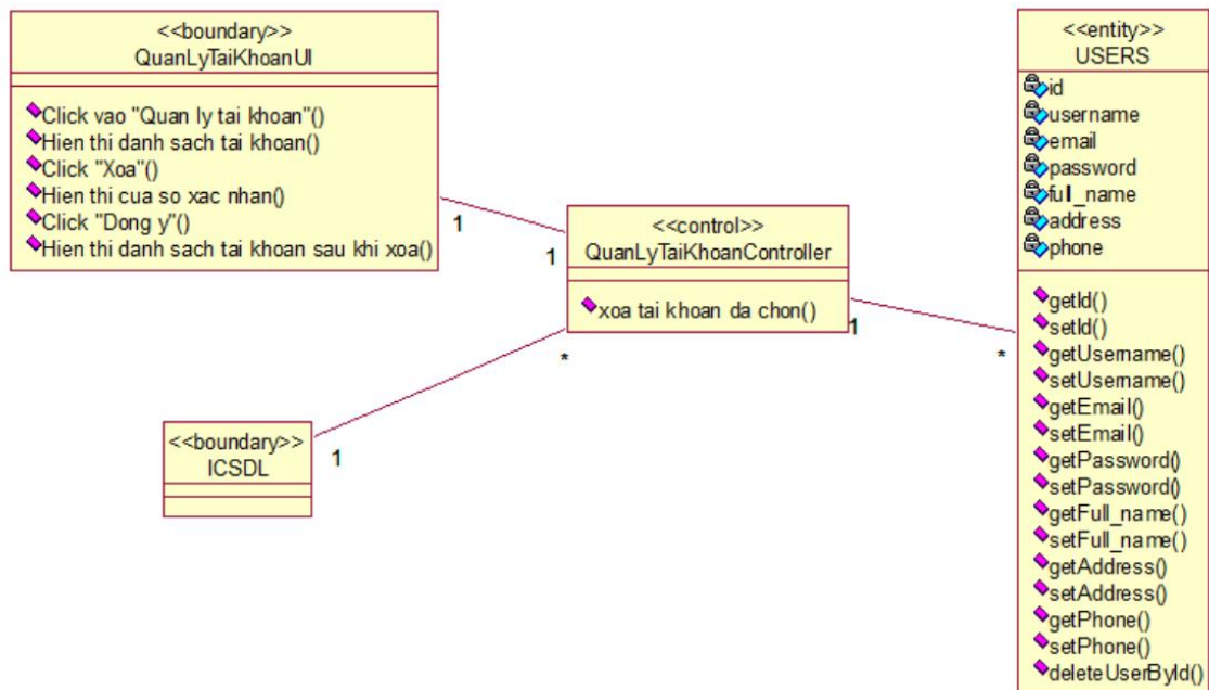
Hình 3.36. Biểu đồ lớp (VOPC) chức năng “Quản lý tài khoản”
