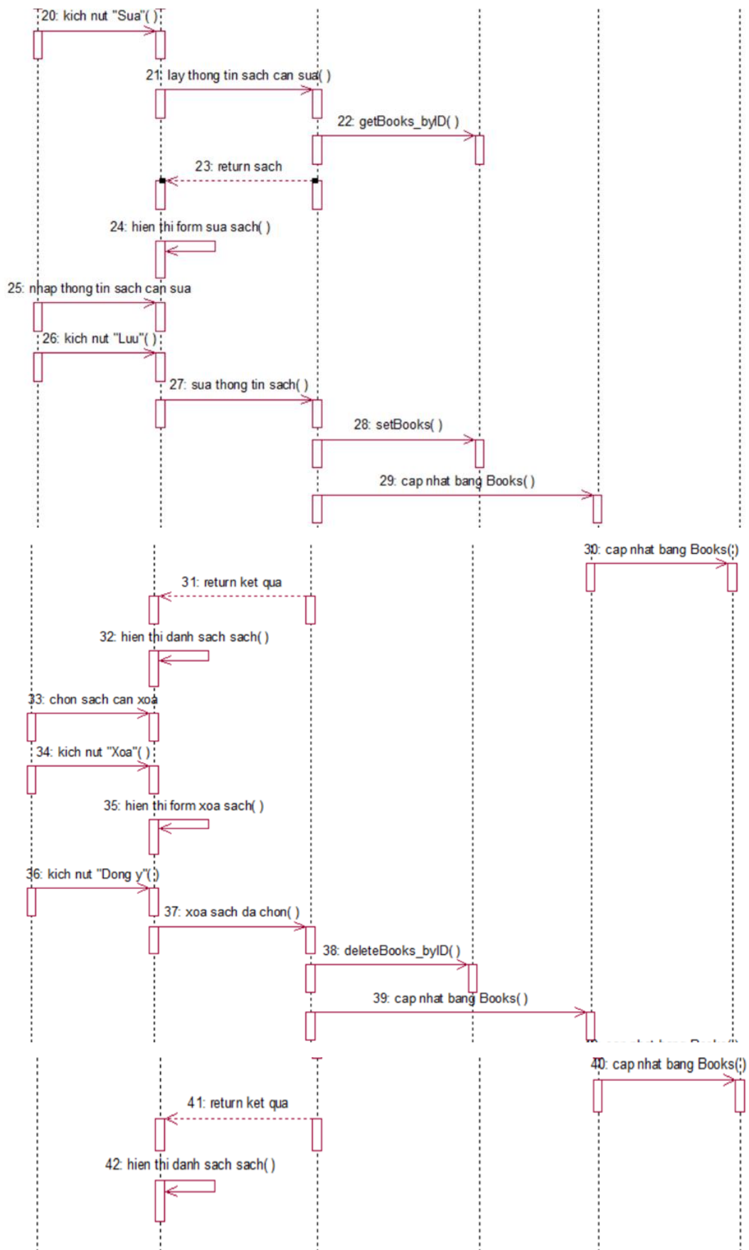
Hình 3.31. Biểu đồ trình tự chức năng “Quản lý sách”
