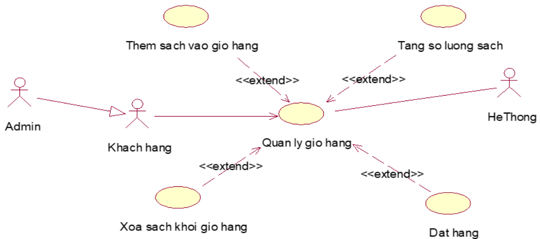
Hình 2.9. Mô hình hóa use case Quản lý giỏ hàng
