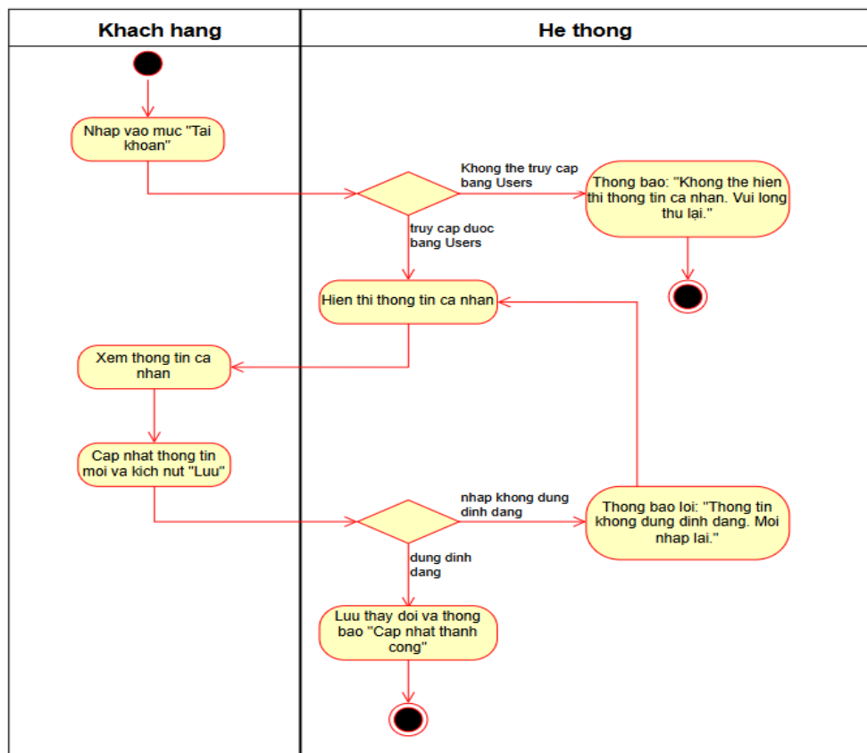
Hình 3.26. Biểu đồ hoạt động chức năng “Quản lý thông tin cá nhân”
