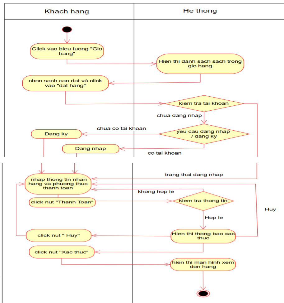
Hình 3.22. Biểu đồ hoạt động chức năng “Đặt hàng”
