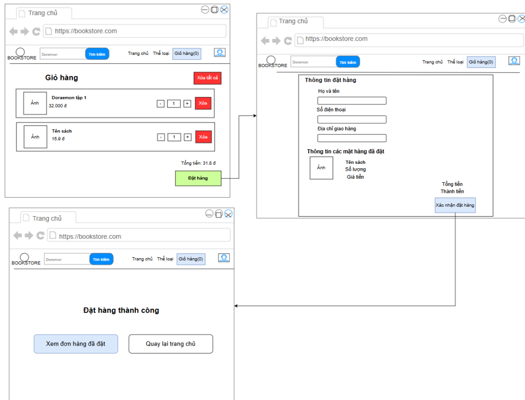
Hình 3.46. Mô phỏng màn hình “Đặt hàng”
