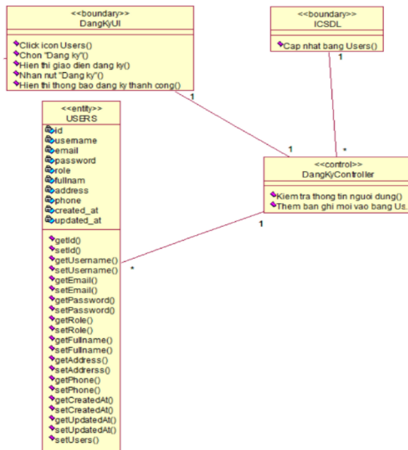
Hình 3.4. Biểu đồ lớp (VOPC) chức năng “Đăng ký”
