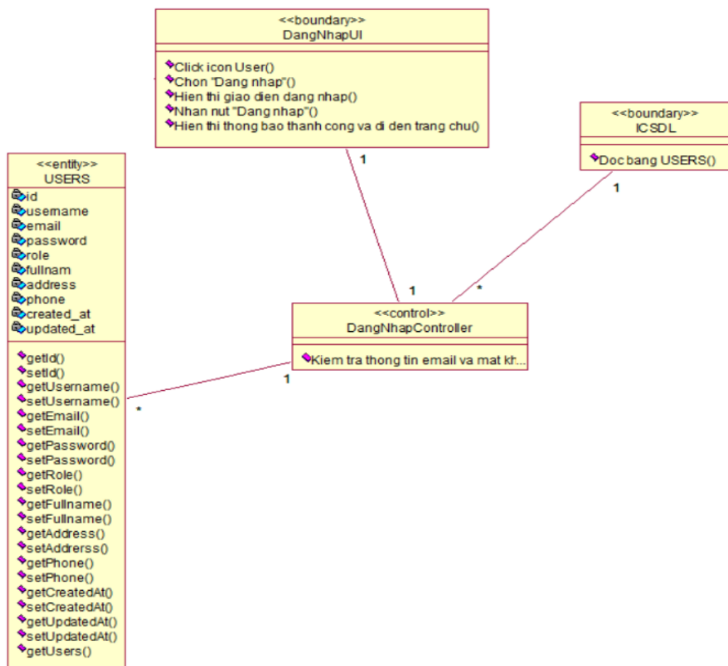
Hình 3.8. Biểu đồ lớp (VOPC) chức năng “Đăng nhập”
